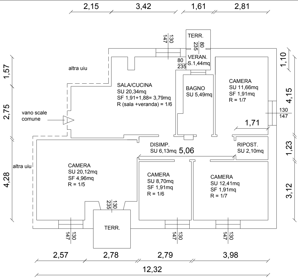
PIANO PRIMO H 3,00ml
