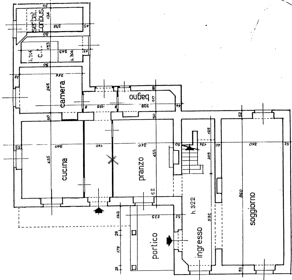
FABBRICATO "D" piano terra
